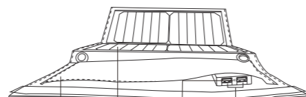
デバイス充電室 ソーラーパネル LED充電インジケター USB充電ポート
