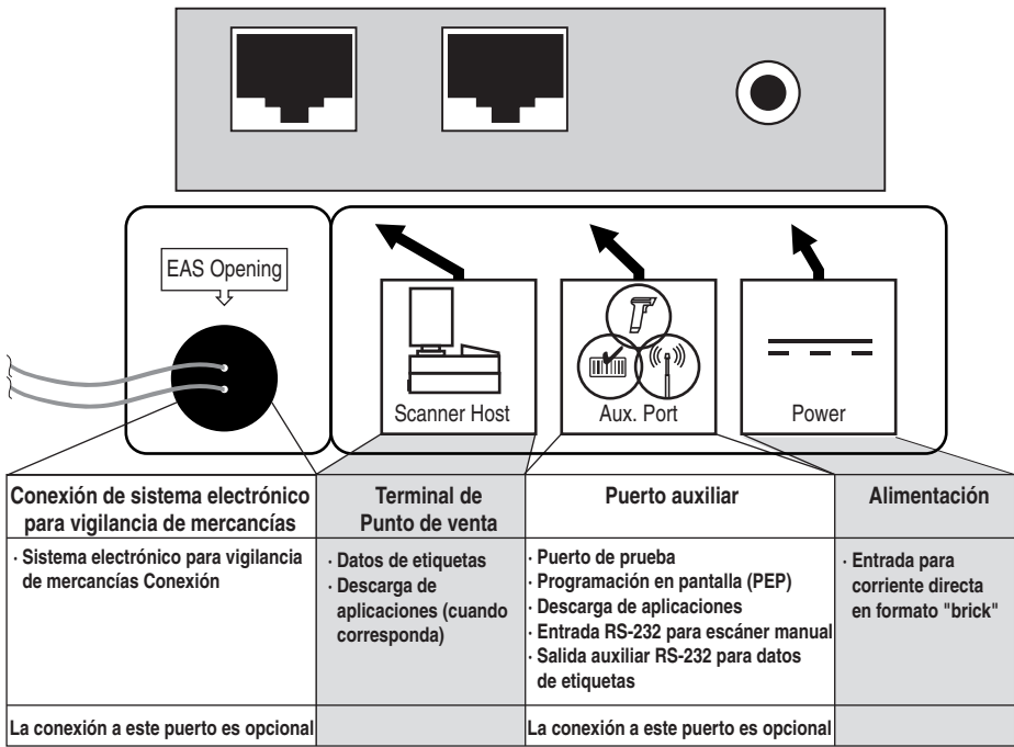
Figure 9. Conexiones
