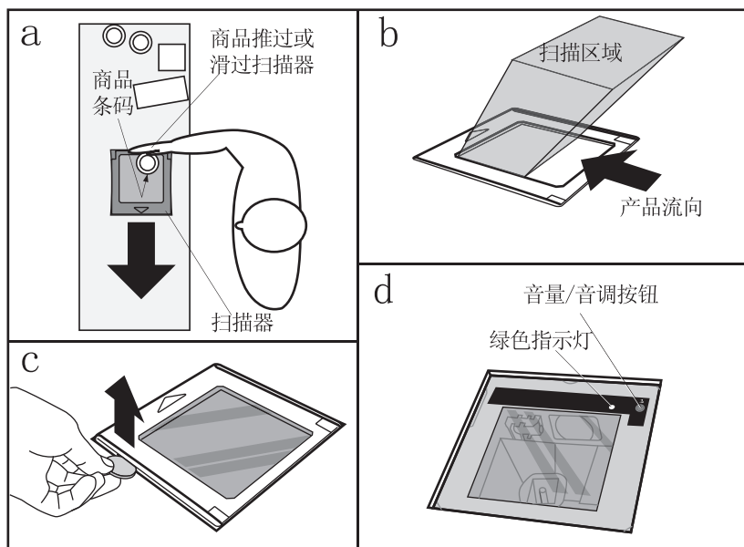
图 14. 操作扫描器
