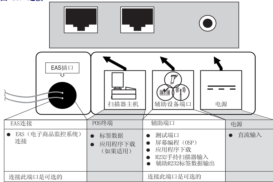
图 13. 连接
