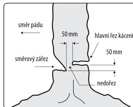
Popis kácení: podřezávání, obr. 11
