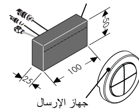
وضع الهوائي
