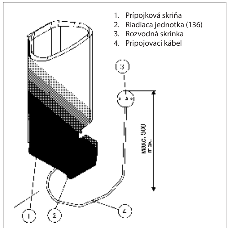
Obrázok 9. Pripojenie kachlí
