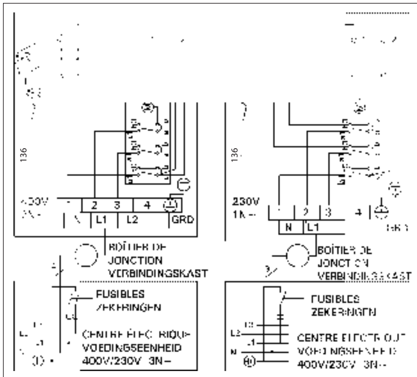
Figure 10. Raccords électriques du poêle (136)
