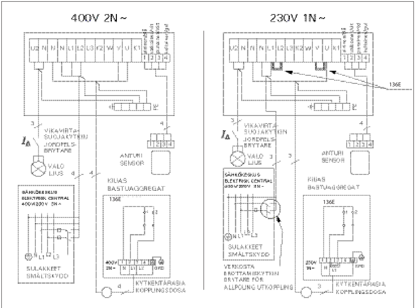
Kuva 12. Ohjauskeskuksen ja kiukaan sähkökytkennät (136E) Bild 12. Elininstallationer av styrcentral och aggregat (136E)
