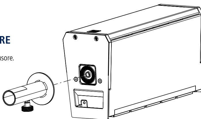
POLE MOUNT KIT per NXL 14-A
