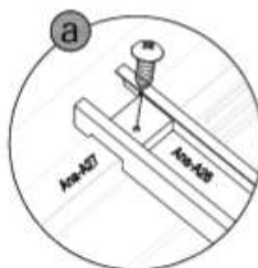
Ana-A26 x2
