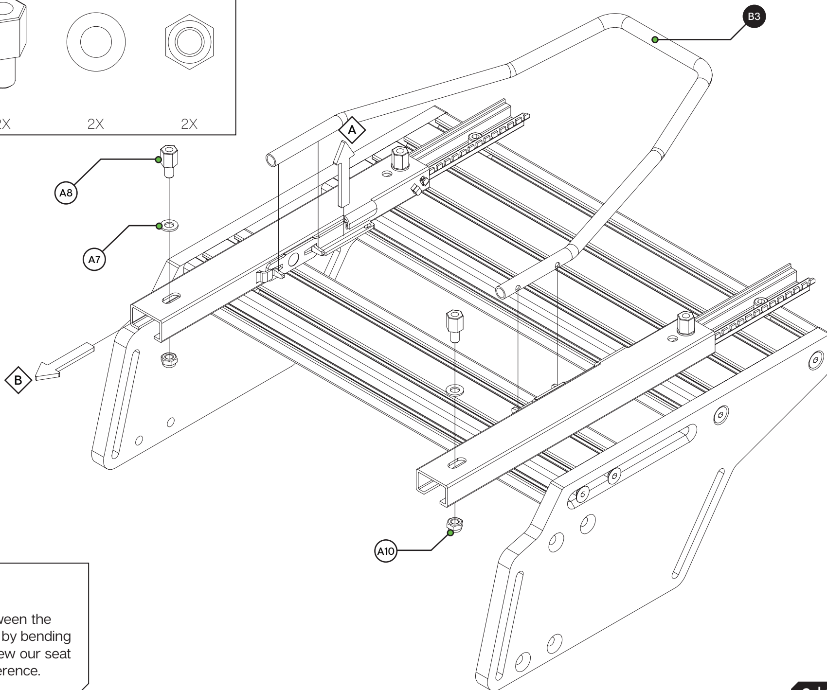
Spacer M8 X 15
