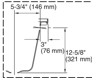
Drain Detail Détails du drain Detalle del desagüe
