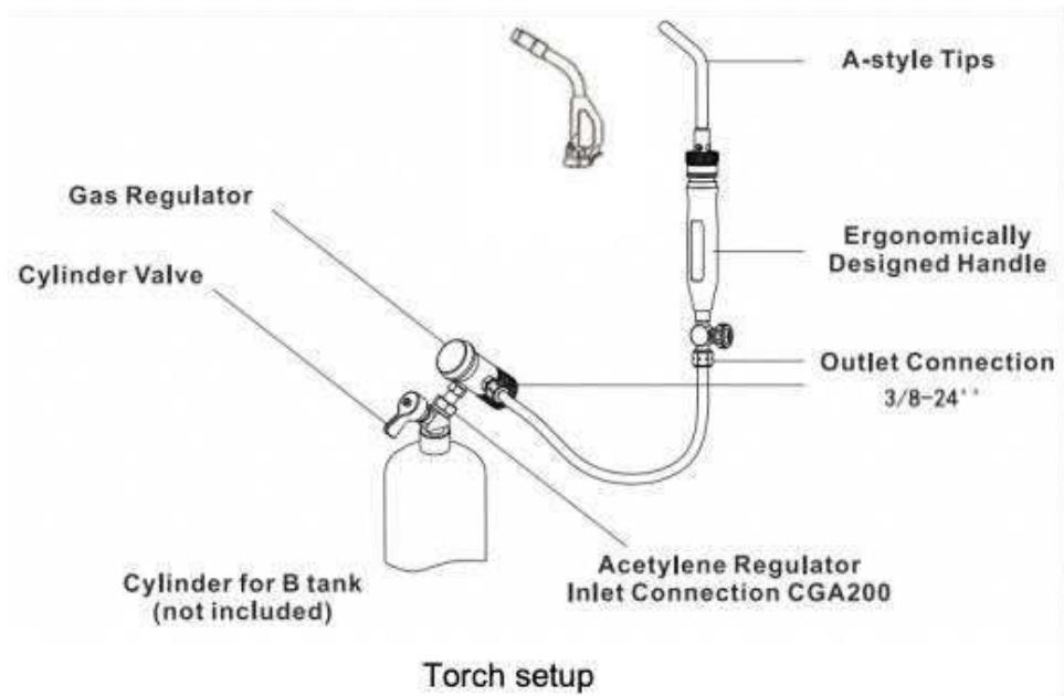
Antorcha configuración
