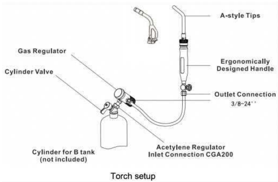
Torcia impostare
