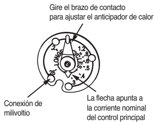
Figura 5. Ajuste del anticipador
