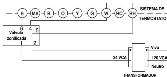
Figura 7. Conexión típica para sistemas de válvula zonificada de 3 cables de solo calor
