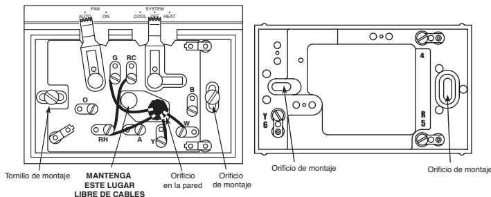
Figura 1. Subbase y placa de pared del termostato
